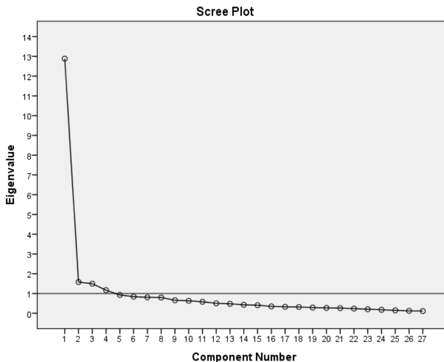
شکل ۱. نمودار اسکری ارزش‌های ویژه عامل‌ها
