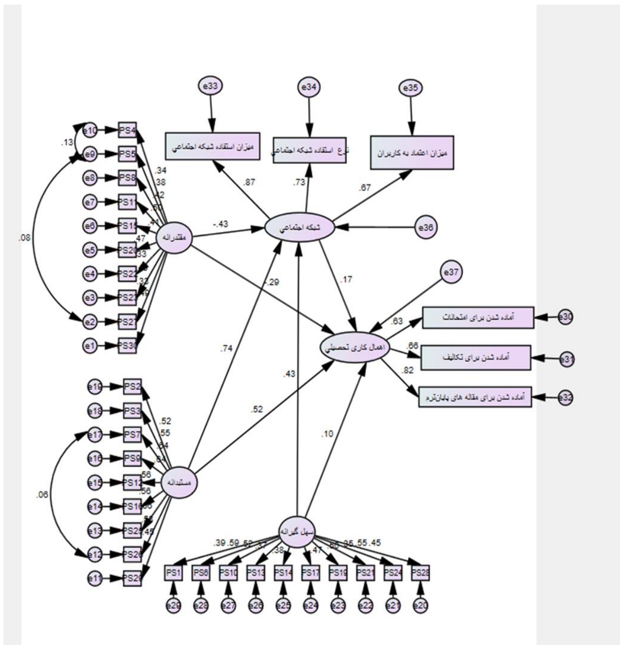
شماره ۱ - مدل ساختاری پژوهش - مدل با ضرایب استاندارد
